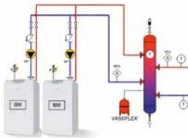
Con botella equilibrado
