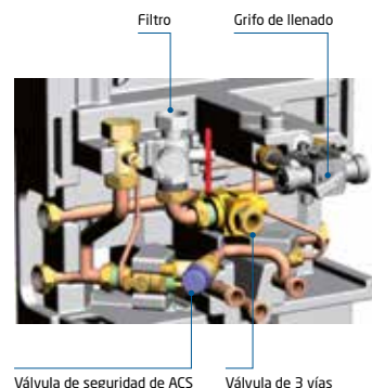
Detalle de los componentes del kit hidráulico
