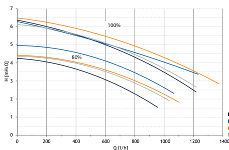
Circulador modulante gama Platinum iPlus
