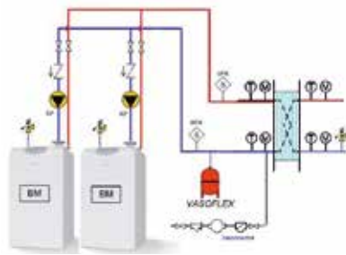
Con intercambiador de placas
