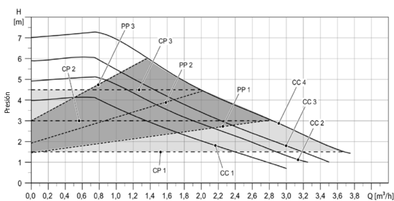
Curvas circulador incluido en los módulos PSG y PSMG
